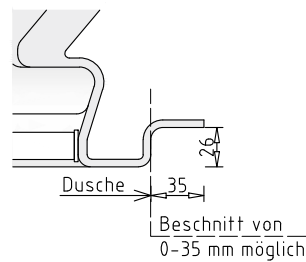
Detail X (seitlicher Flansch)
