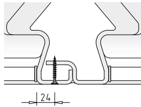
Detail Befestigung Dusche/Dusche
