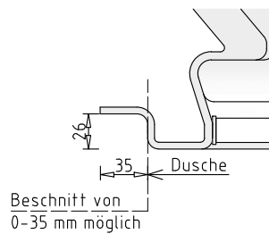
Detail X (seitlicher Flansch)
