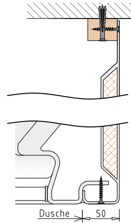
Detail GFK-Seitenblende
