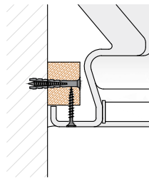
Detail Wandanschluss
