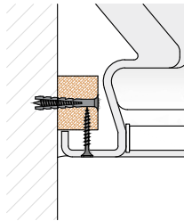
Detail Wandanschluss
