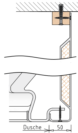
Detail GFK-Seitenblende
