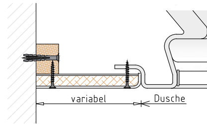
Detail GFK-Frontblende oder bauseitige Beplankung
